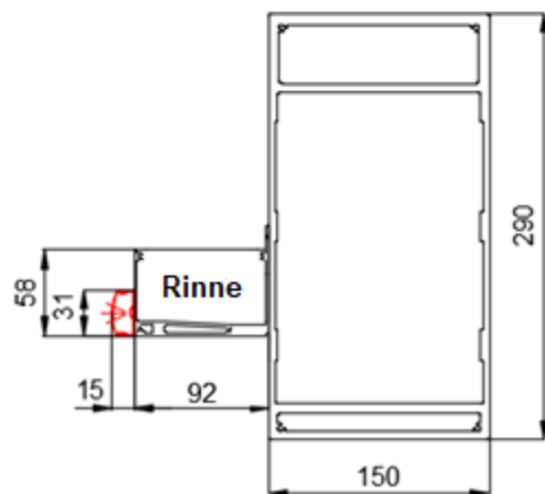
Seitliche Strebe
