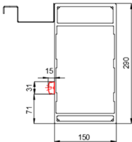
Vorder/Hintere Strebe
