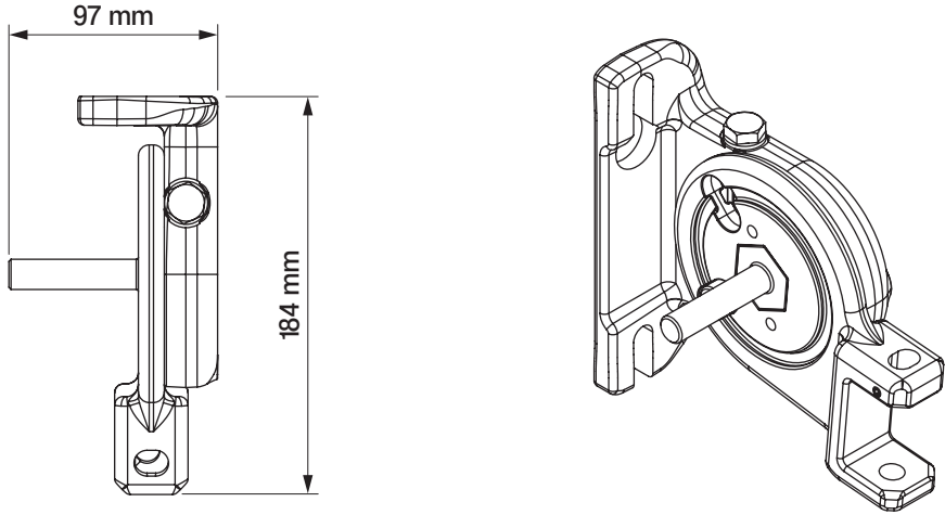
uchwyt ścienna-sufitowy prawy malta
