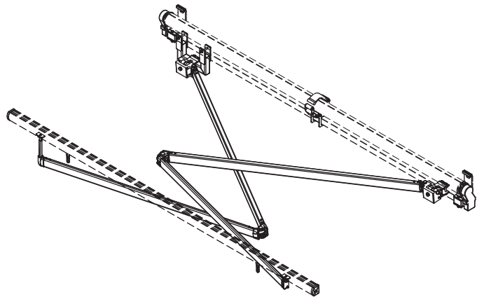
ramiona krzyżowa w opcji
