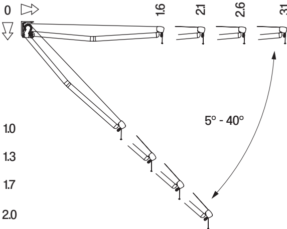
kąt pochyłu
