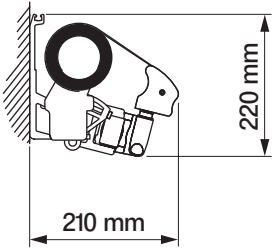
montaż do ściany
