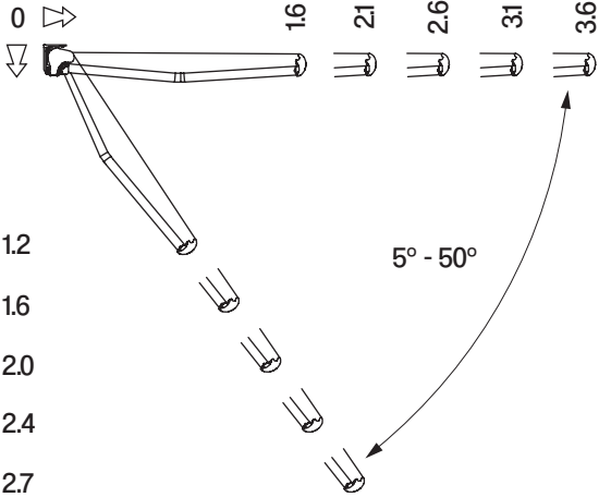
kąt pochyłu
