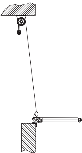
mocowanie do haka ramienia
