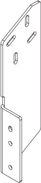
uchwyt dachowy
