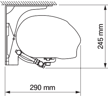
montaż do sufitu
