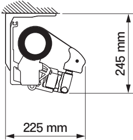
montaż do sufitu
