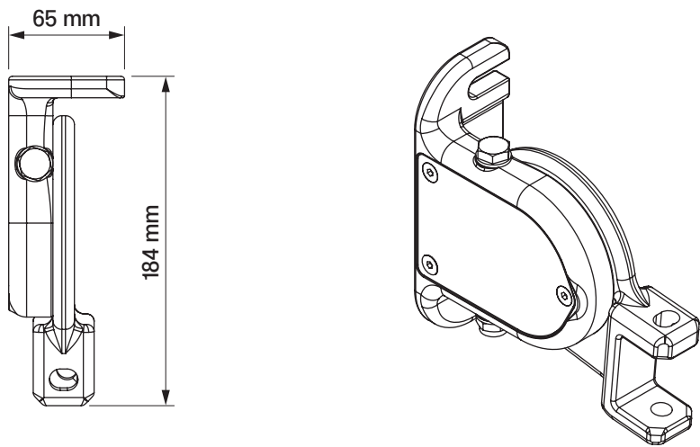
uchwyt ścienna-sufitowy lewy malta
