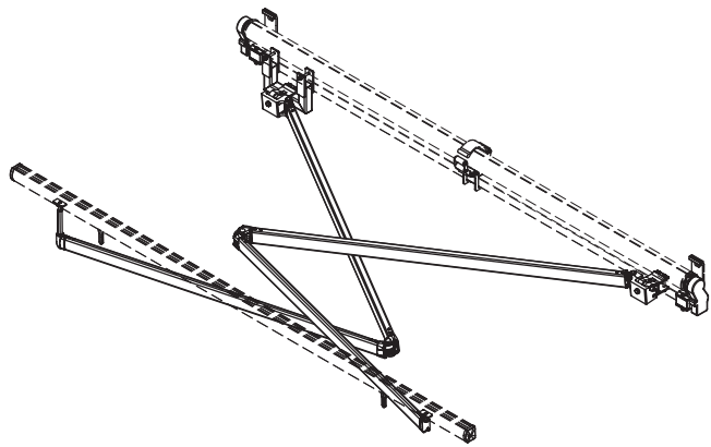
ramiona krzyżowa w opcji
