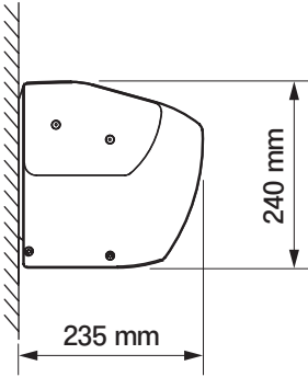
montaż do ściany
