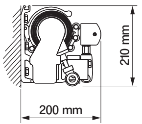
montaż do ściany
