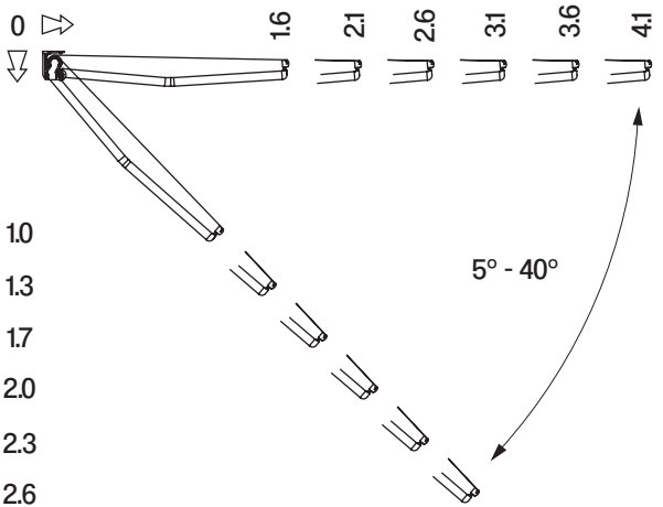
kąt pochyłu
