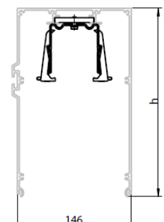
Przekrój kasety Cube
