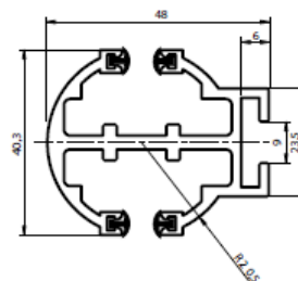
Prowadnica okrągła podwójna
