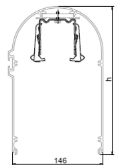
Przekrój kasety Oval
